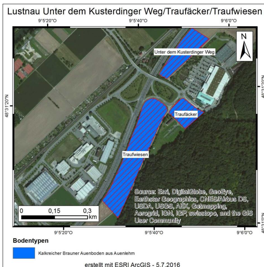
Abbildung 8: Bodentypen im Bereich der geplanten Gewerbebestandorte "Unter dem Kusterdinger Weg", „Traufäcker“ und „Traufwiesen“
